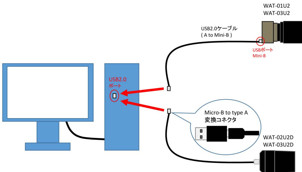
図 1 Watec USB Camera – PC 接続図
