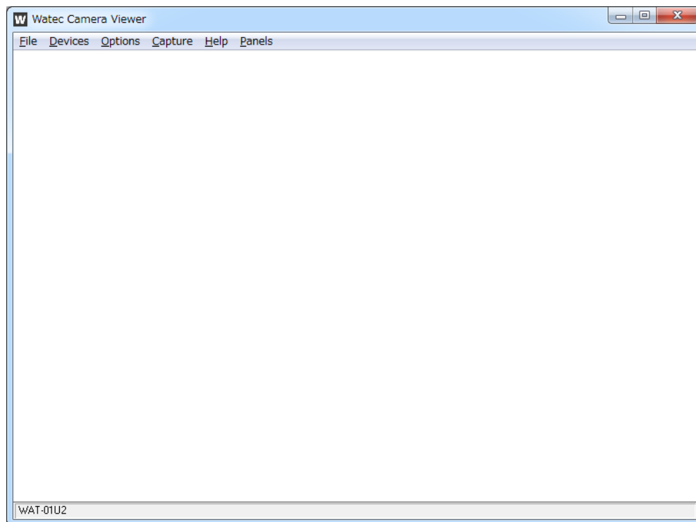
図 2 WatecCameraViewer の外観
